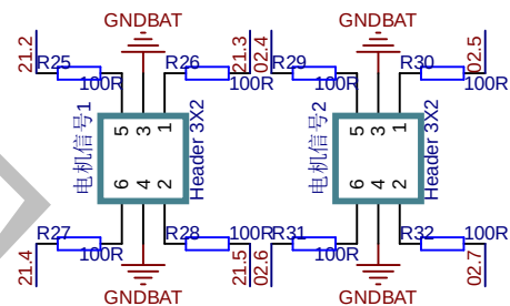
电机接口
